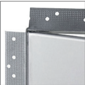
PFI-GYP Panneau d'accès isolé homologué contre le feu avec cadre perforé pour gypse
